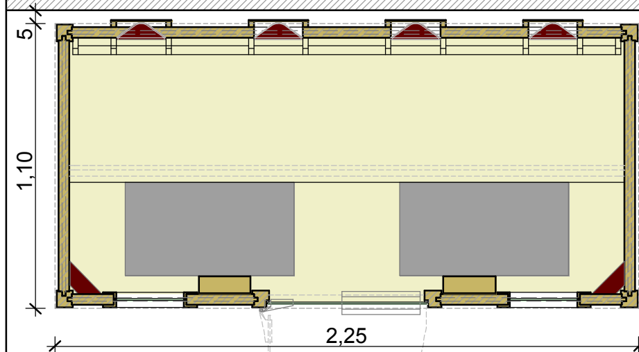
alaprajz
