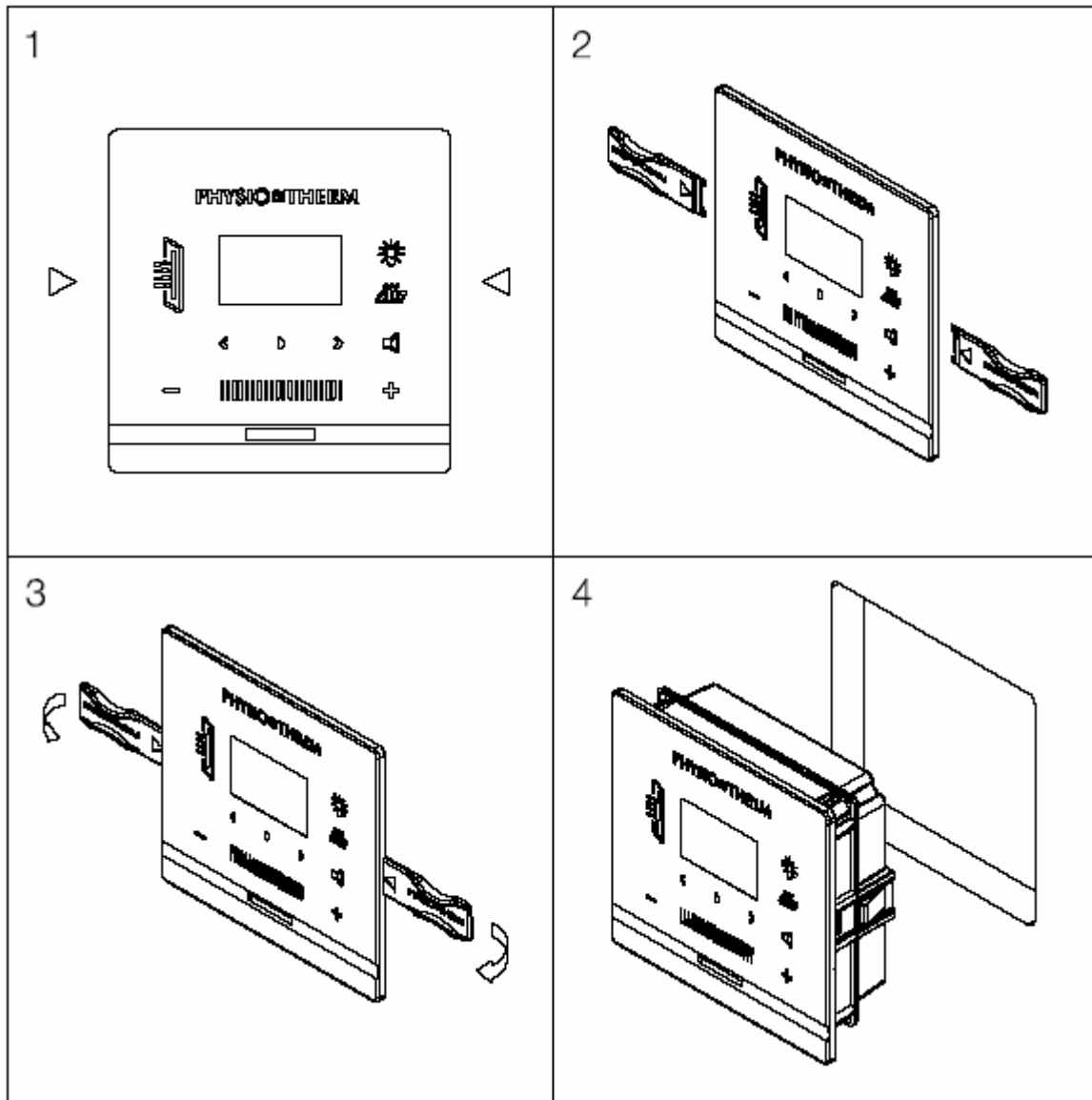
12. sz. ábra: Kezelőfelület kiserelése
