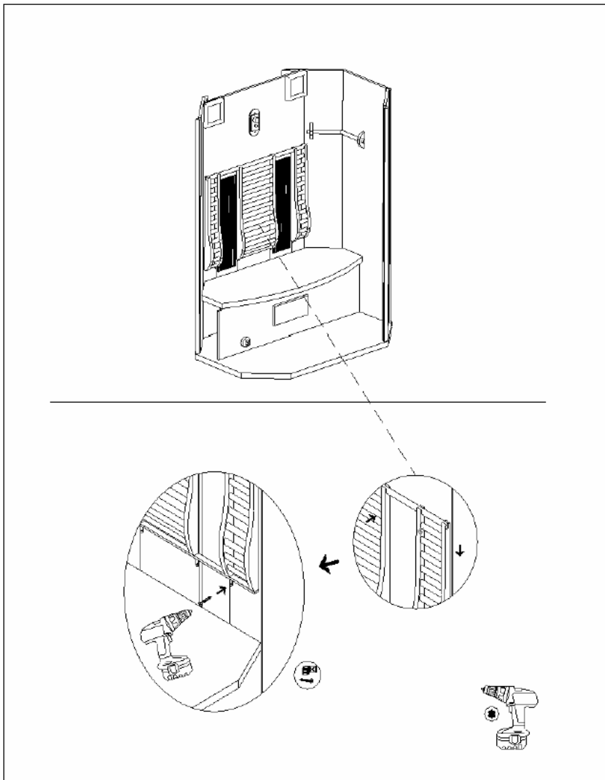
11. sz. ábra: Háttámla szerelése
