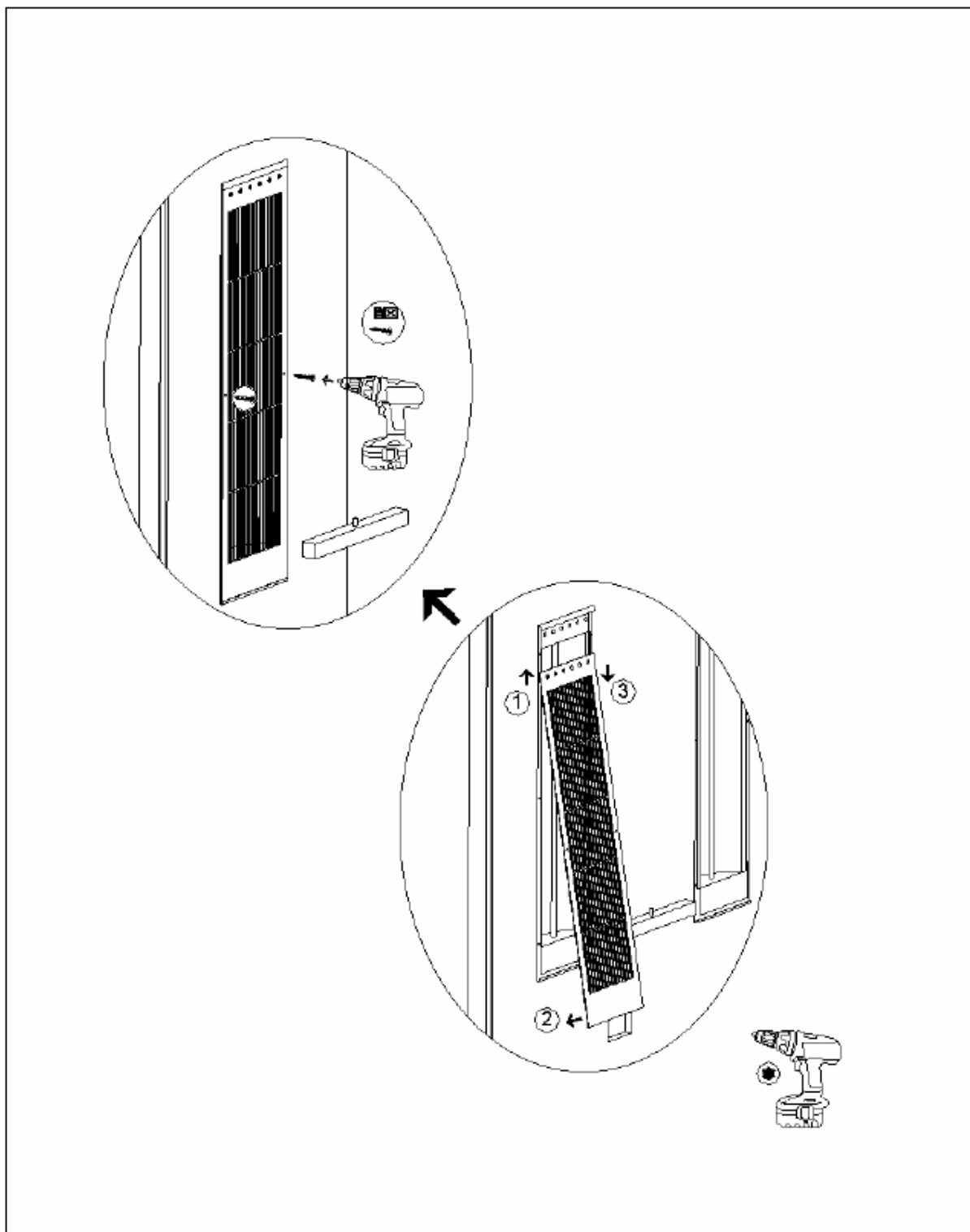
10. sz. ábra: takarórács szerelése tisztítás után
