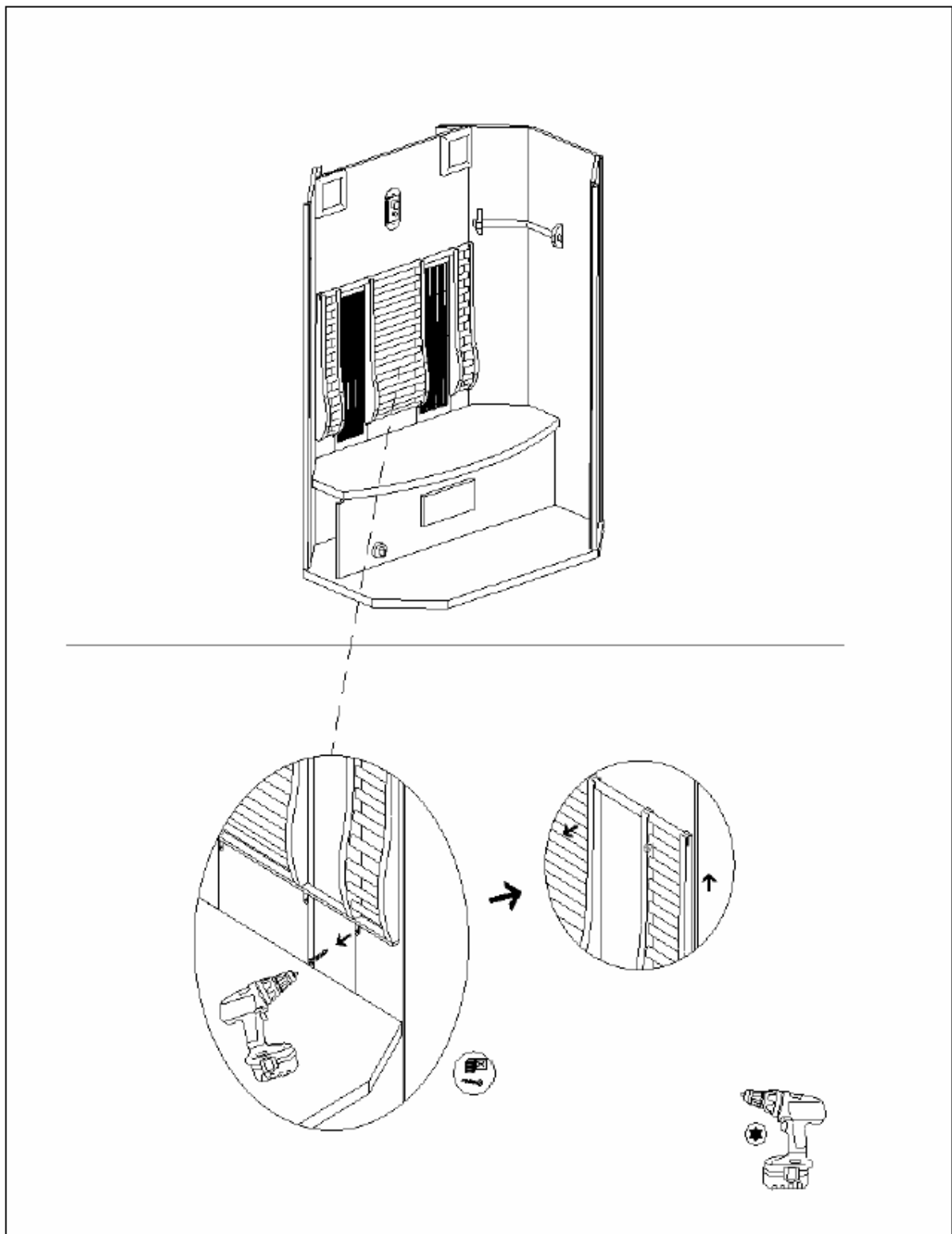
8. sz. ábra: háttámla leszerelése
