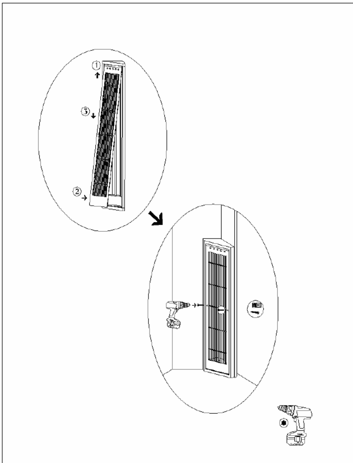
7. sz. ábra: Takarórács szerelése tisztítás után
